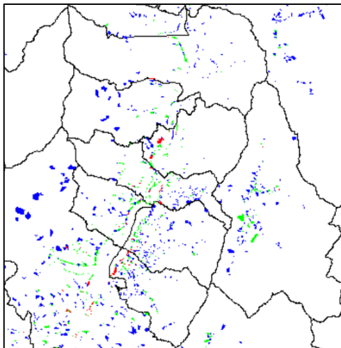
南海トラフ巨大地震（基本ケース） の土砂災害危険度（急傾斜地崩壊危険箇所 ・山腹崩壊危険地区）
