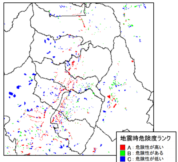
南海トラフ巨大地震（陸側ケース） の土砂災害危険度（急傾斜地崩壊危険箇所・ 山腹崩壊危険地区）
