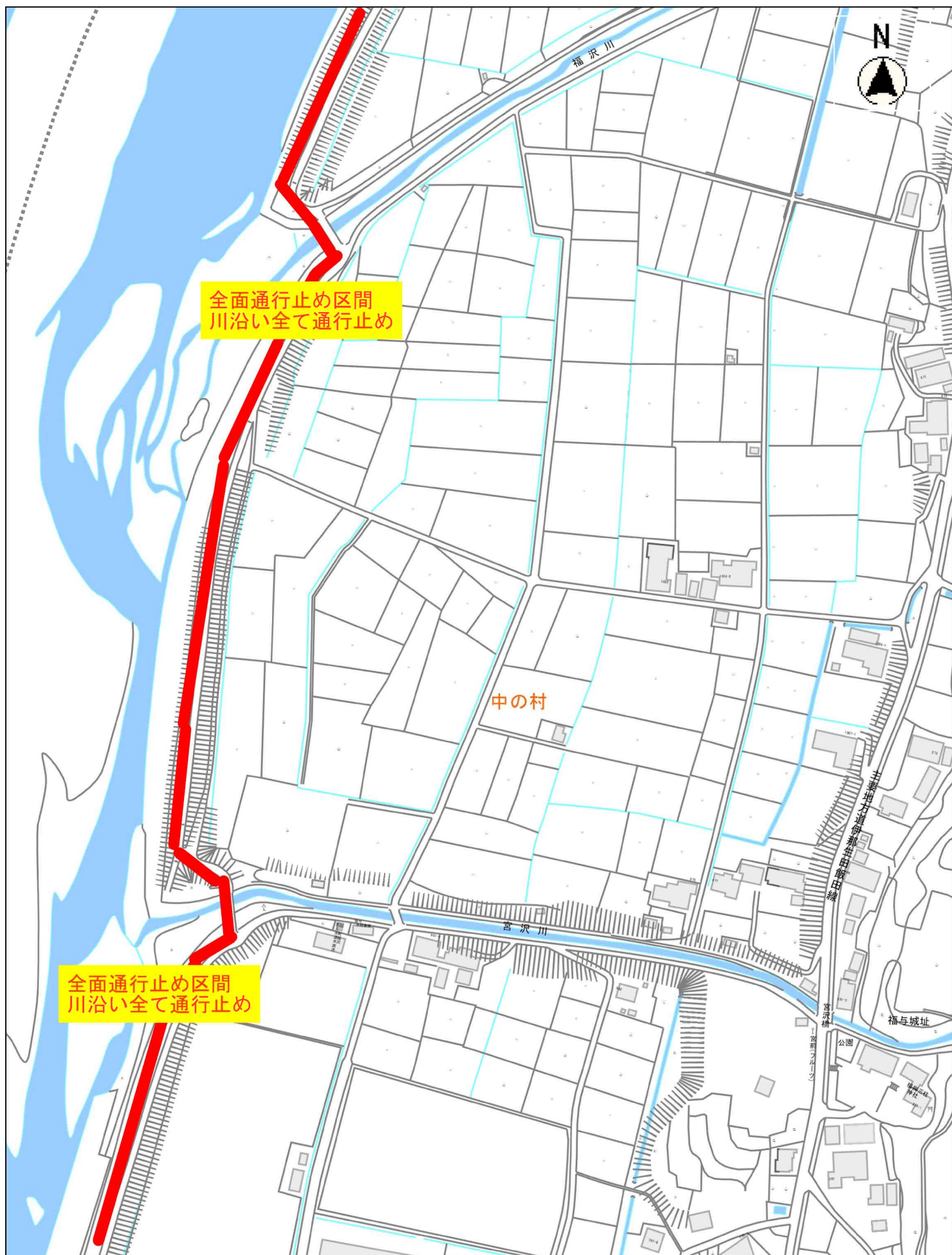
交通規制図 5 縮尺 1 : 2500 20 10 0 10 20 30 40 50 60 70 80 90 100 110 120 130 140 150 160
